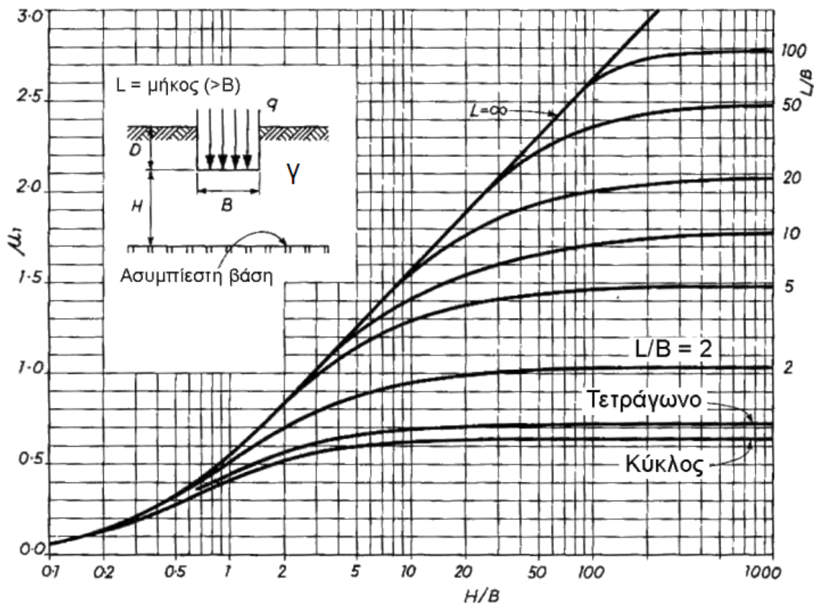
Σχήμα σελ. 6.27 Νομογραφήματα \mu_0 και \mu_1 για τον υπολογισμό καθιζήσεων σε αργιλικά εδάφη με τη μέθοδο Janbu et al. (1956)
