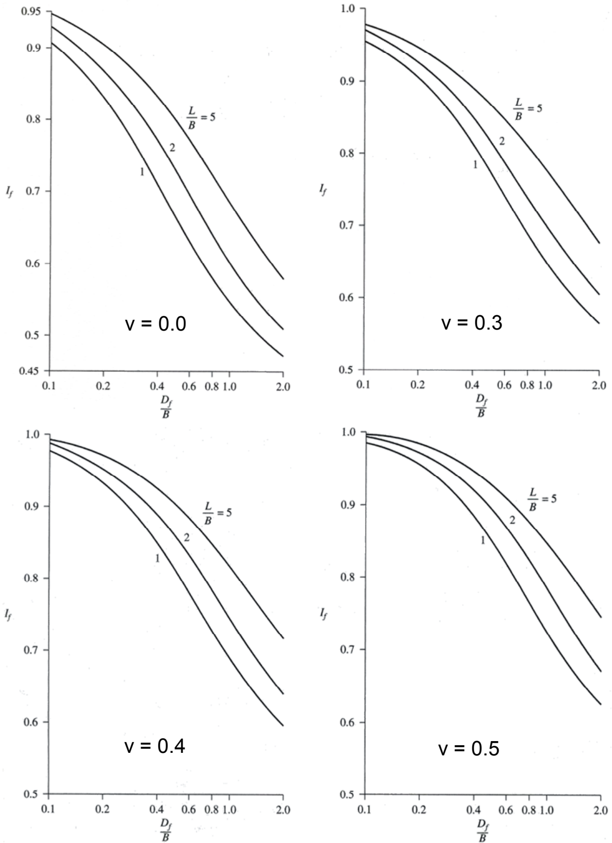
Σχήμα σελ. 6.20 Νομογραφήματα για τον υπολογισμό του I_F
