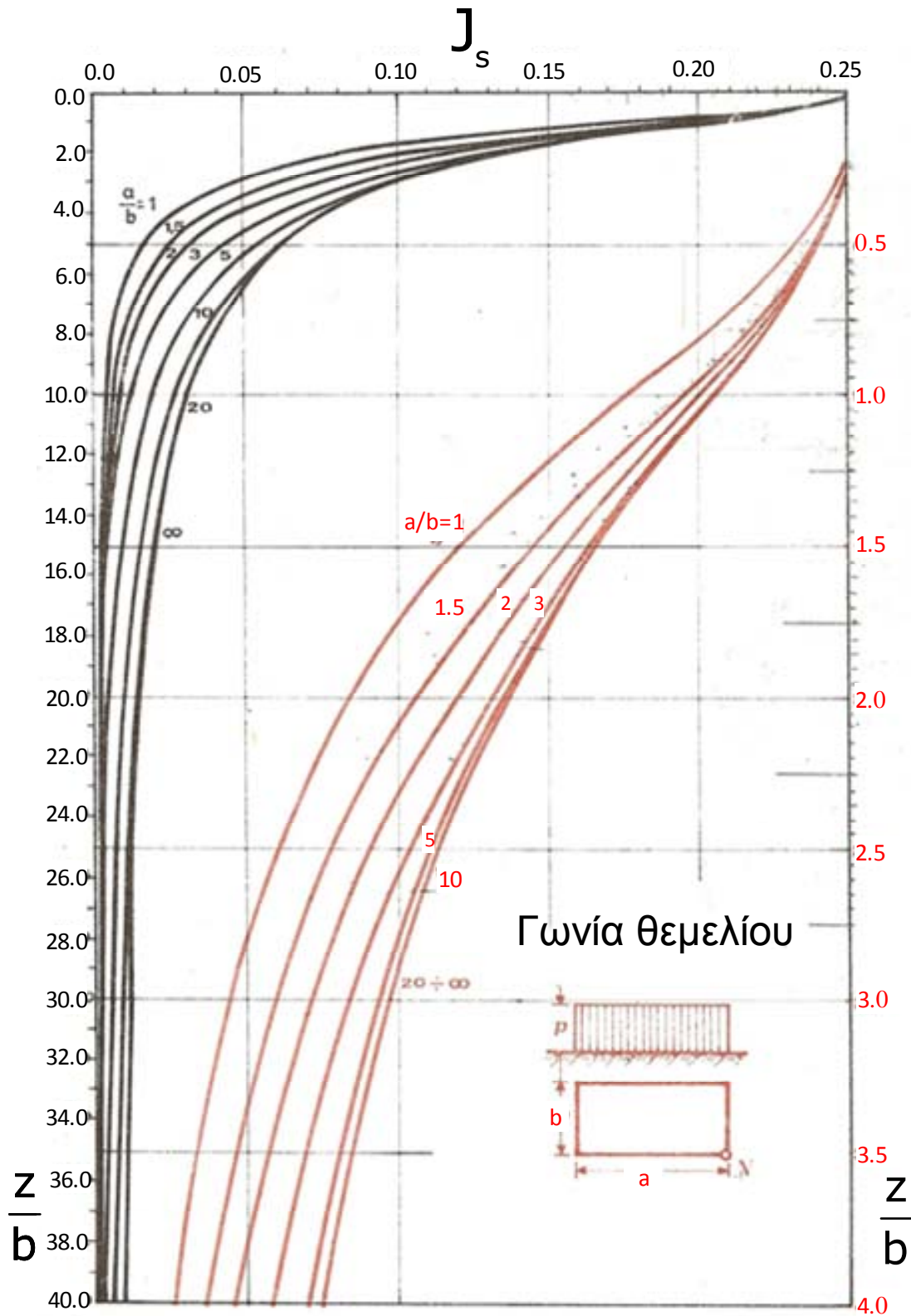
Σχήμα σελ. 6.5 Τάσεις επιφόρτισης στη γωνία πεδίου (στο σχήμα B=b και L=a ).
