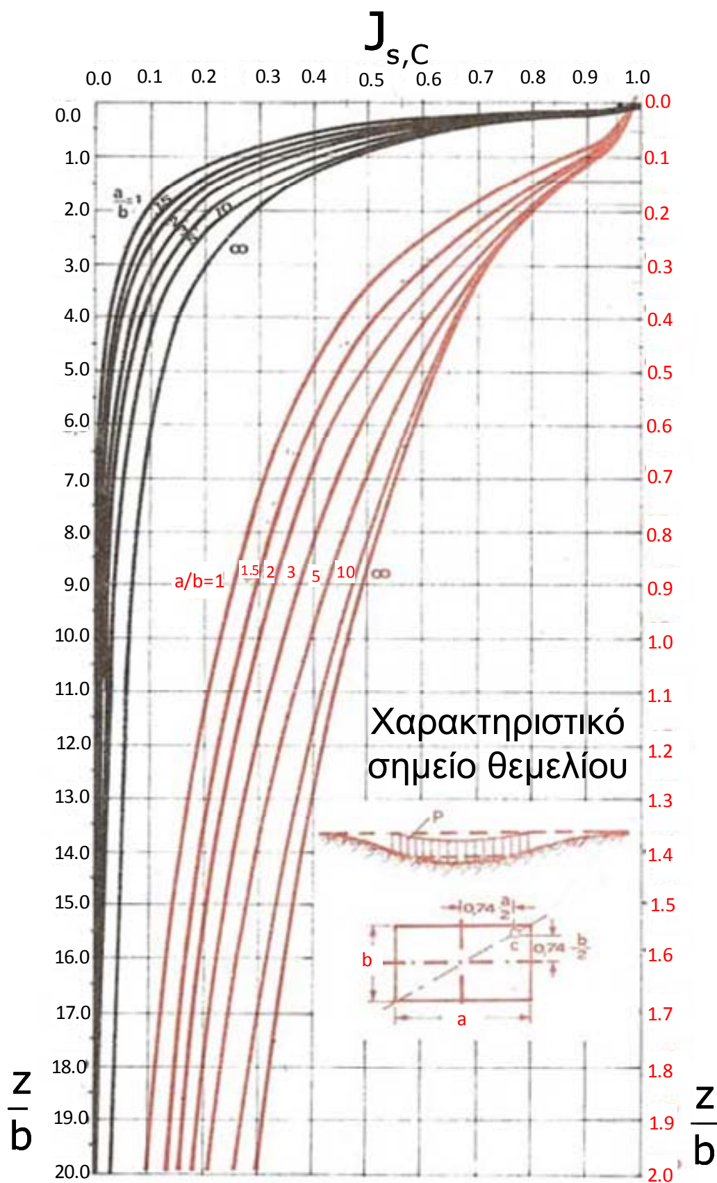
Σχήμα σελ. 6.6 Τάσεις επιφόρτισης στο χαρακτηριστικό σημείο πεδίου (στο σχήμα B=b και L=a ).
